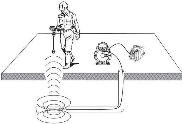
Рис. 27 – Местонахождение зонда microReel
